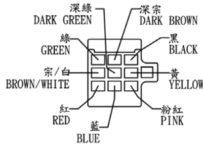
"A" 詳圖
